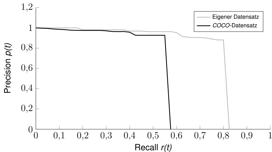
Abbildung 4.5: Precision-Recall Kurven des entwickelten SSD MobileNet V2 Netz.
