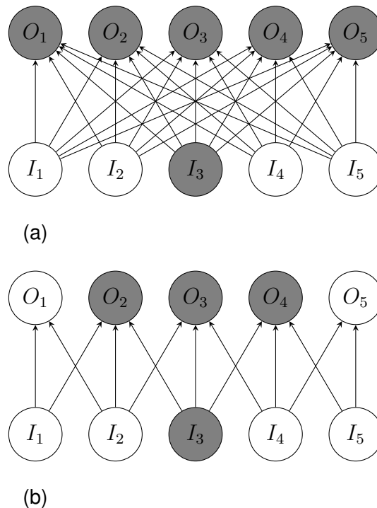
Abbildung 2.8: (a) Abbildung zweier Schichten eines herkömmlichen, künstlichen, neuronalen Netzes. Die Flussrichtung der Bildinformationen ist mit Pfeilen angedeutet. Horizontal ausgerichtete Kreise stellen eine Schicht dar. Graue Kreise zeigen Neuronen, die voneinander abhängig sind. (b) Grundlegende Darstellung zweier Schichten eines Faltungsnetzes. Es gelten dieselben Darstellungsprinzipien wie in Abbildung a [13].
