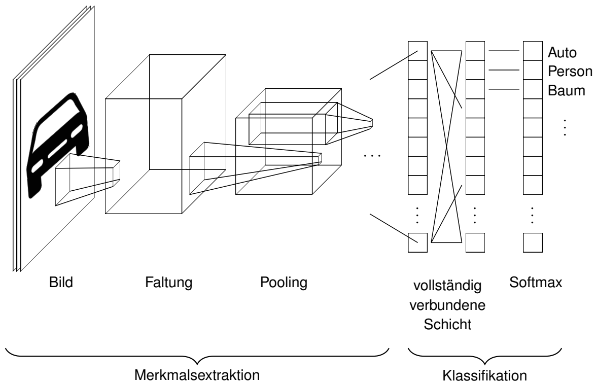
Abbildung 2.6: Prinzipdarstellung eines Faltungsnetzwerks. Fortsetzungen werden mit drei aufeinander folgenden Punkten gekennzeichnet. Durch rechteckige Formen werden Schichten dargestellt. Angedeutet durch Pyramidenstümpfe werden Prozesse der Faltung und des Poolings dargestellt. Darstellung adaptiert aus [24, 25].
