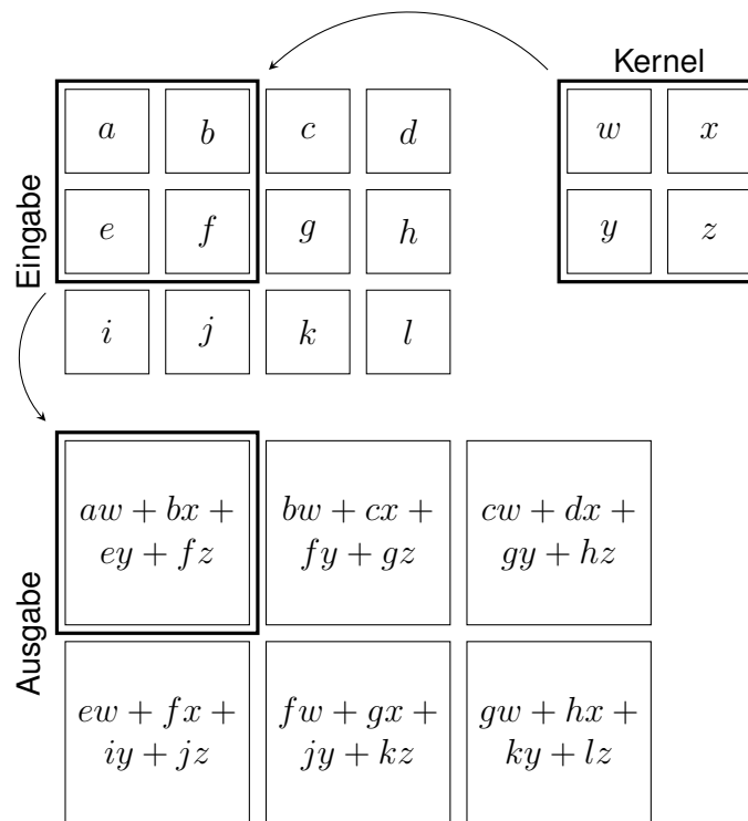
Abbildung 2.7: Prinzipielle Darstellung des Faltungsprozesses. Mit einem Quadrat umrandete Buchstaben stellen Daten wie zum Beispiel einen Pixel dar. Der Kernel fasst in dieser Abbildung beispielsweise vier Daten zu einer Information zusammen und gibt diese aus. Adaptiert aus [13].
