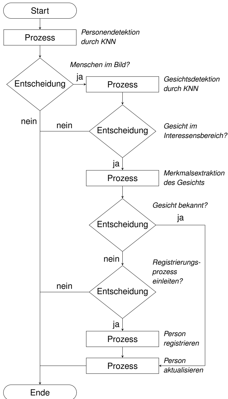
Abbildung 3.8: Prozessablaufplan der Personenerkennung. Der Start sowie das Ende des Programms sind als Boxen mit Abrundungen dargestellt. Rechtecke zeigen Prozesse und Parallelogramme deuten eine Entscheidung im Programmablauf an. Die Flussrichtung der entsprechenden Informationen wird durch Pfeile präsentiert.
