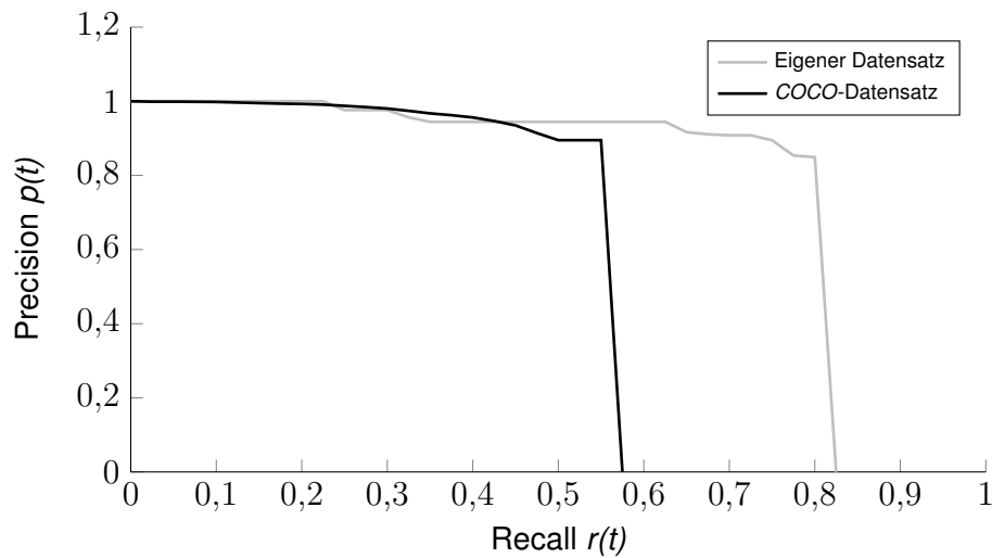
Abbildung 4.6: Precision-Recall Kurven eines MobileNet V2 SSDLite Netzes [61].
