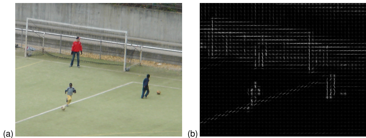
Abbildung 2.4: (a) Foto von drei spielenden Personen [21]. (b) Darstellung der Gradienten, die durch einen HOG erzeugt worden sind. Der weiße Farbverlauf deutet die Richtung der analysierten Konturen an. Die Analyse erfolgte mit Bild a [21].
