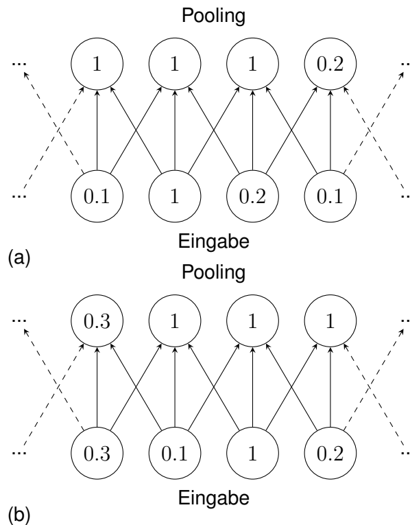
Abbildung 2.9: (a) Beispielhafter Poolingprozess. Die Zahlenwerte deuten Bildinformationen als Fallbeispiel an. (b) Es gelten dieselben Darstellungsprinzipien wie in Abbildung (a). Die Eingangsdaten wurden hierbei um ein Neuron nach rechts versetzt. [13]
