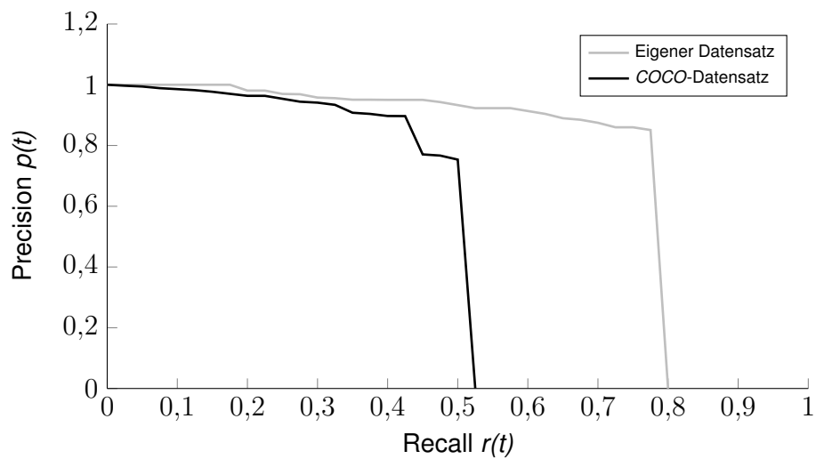
Abbildung 4.7: Darstellung der Precision-Recall Verläufe des entwickelten MobileNet V2 SSDLite Netz.
