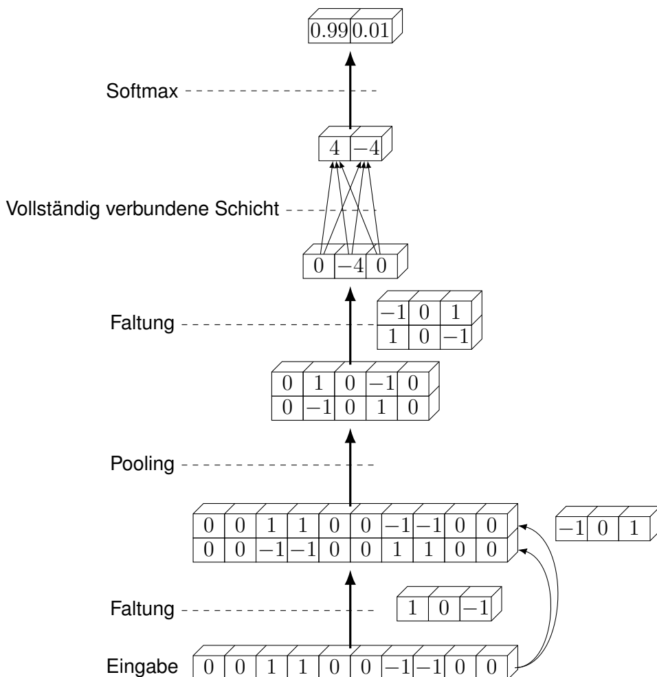
Abbildung 2.10: Fallbeispiel eines Faltungsnetzwerks. Dreidimensional dargestellte Boxen stellen Datenpunkte dar und bilden in der horizontalen Anordnung jeweils eine Schicht. Die Prozesse der Faltung und des Poolings sind beispielhaft dargestellt. Die Flussrichtung der Bildinformationen ist durch Pfeile gekennzeichnet. [26]
