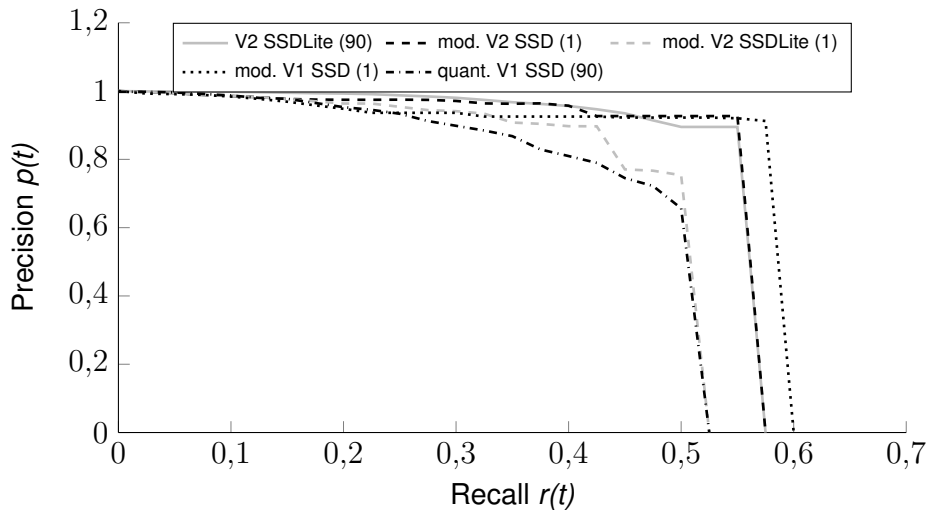
Abbildung 4.10: Precision-Recall Kurven aller MobileNet Netze in Anwendung auf den COCO -Datensatz. Die Abkürzungen mod. und quant. stehen für modifiziert und quantisiert .
