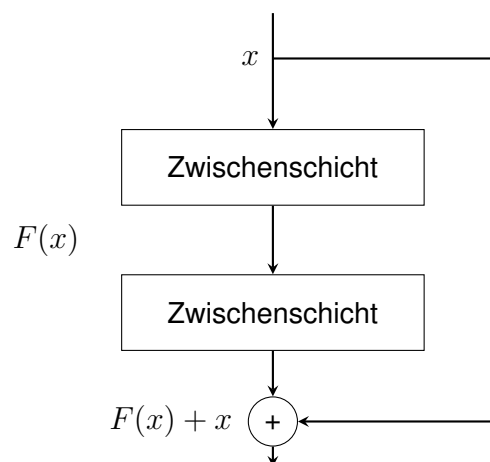
Abbildung 2.11: Markantes Merkmal eines ResNets . Die Flussrichtung der Bildinformationen ist als Pfeil dargestellt. Adaptiert aus [30].
