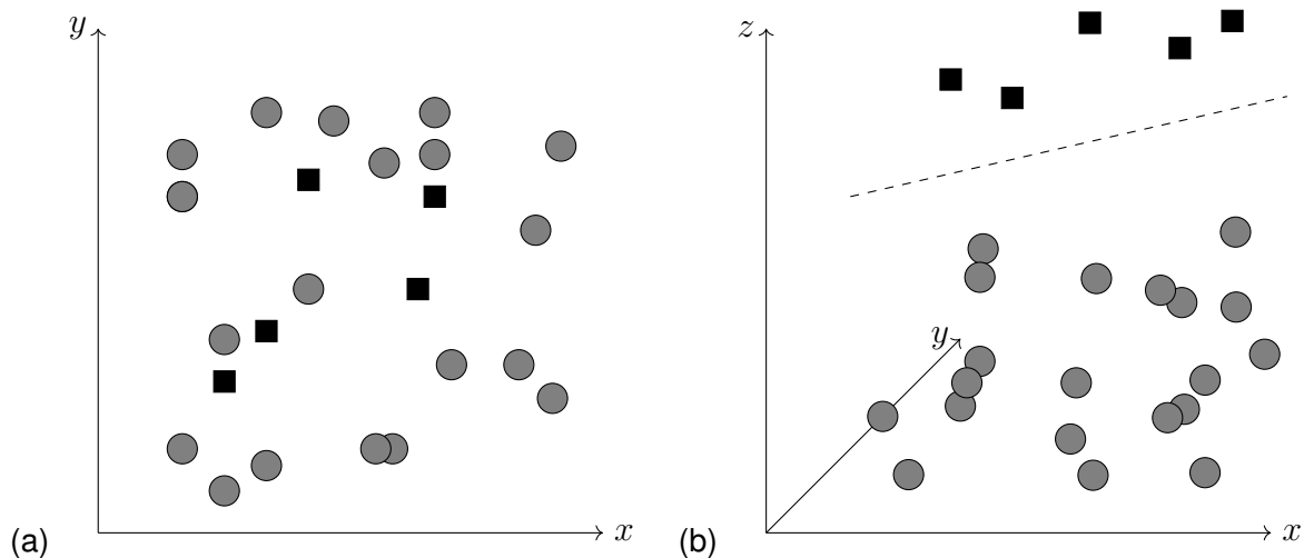
Abbildung 2.5: (a) Abbildung von möglichen, Objektklassen im zweidimensionalen Raum. Die Formen stellen jeweils Klassen dar, wie zum Beispiel die Klassen Hund und Person. (b) Darstellung der in a gezeigten Objektklassen im dreidimensionalen Raum. Die gestrichelte Linie deutet eine lineare Trennung an.
