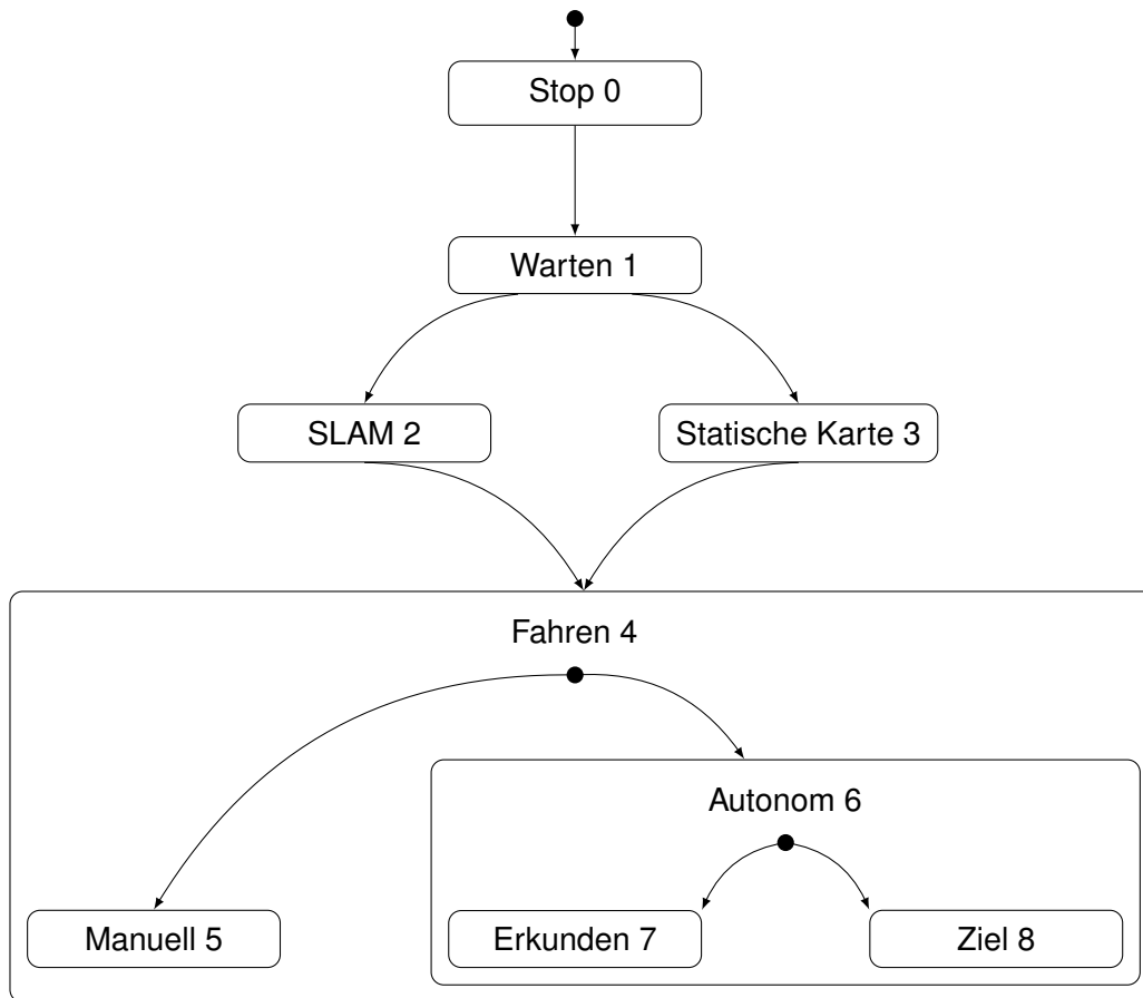
Abbildung 3.9: Konzept eines hierarchischen Zustandsautomaten in Form eines UML-Diagramms. Zustände sind als Boxen mit Abrundungen dargestellt. Ineinander verschachtelte Zustände erben Funktionen von dem jeweils größeren Zustand. Pfeile deuten mögliche Transitionen an. Startzustände werden durch schwarze Punkte gezeigt.
