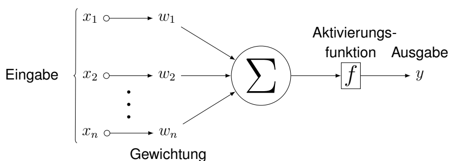
Abbildung 2.1: Darstellung der prinzipiellen Funktion eines Neurons in einem neuronalen Netz. Drei aufeinander folgende Punkte deuten eine Fortsetzung an. [11]
