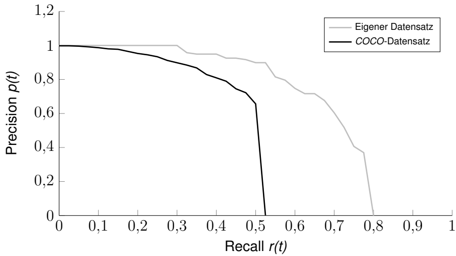
Abbildung 4.3: Gegenüberstellung der Precision-Recall Kurven eines quantisierten SSD MobileNet V1 Netzes [60].
