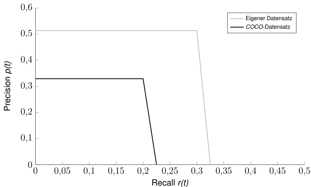
Abbildung 4.1: Precision-Recall Kurven der HOG-SVM Kombination. [59]
