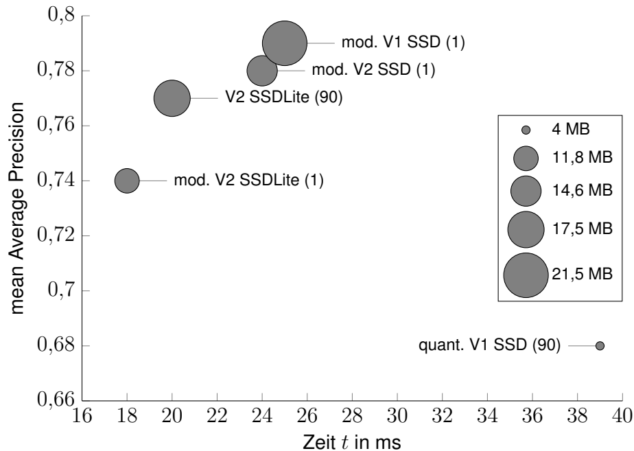
Abbildung 4.11: Vergleich aller untersuchten MobileNet Architekturen. Das Diagramm stellt die mean Average Precision aufgetragen über die gemessene Rechenzeit dar. Gezeigt ist der Test auf dem integrierten Rechner des ALFs in Anwendung auf den eigenen Datensatz.
