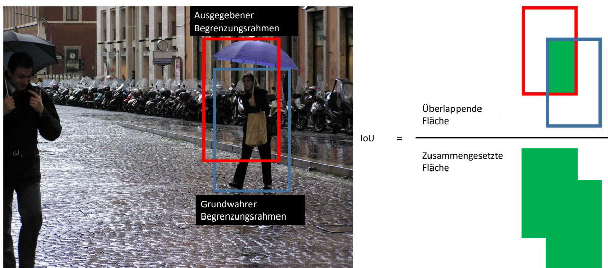
Abbildung 2.3: Darstellung der Ermittlung eines IoU -Werts. Der vertikale Strich auf der rechten Seite der Abbildung stellt einen Bruchstrich dar. Adaptiert aus [18].
