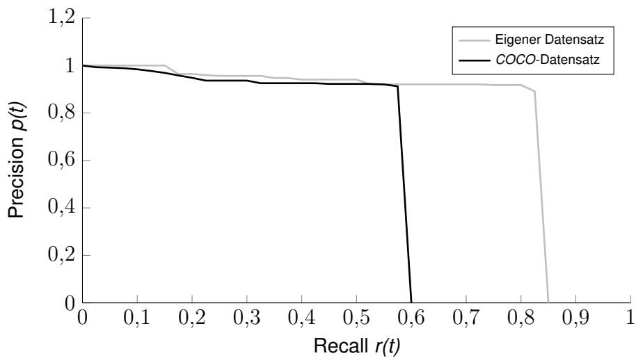
Abbildung 4.4: Precision-Recall Kurven des entwickelten MobileNet V1 SSD Netzes.
