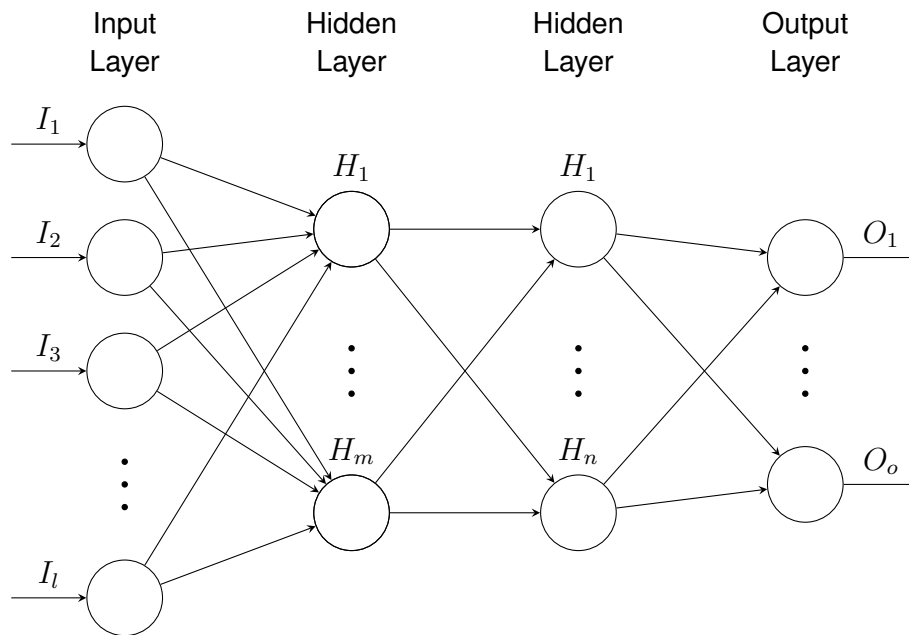
Abbildung 2.2: Prinzipielle Darstellung eines künstlichen, neuronalen Netzwerks. Neuronen werden als Kreise dargestellt. Drei aufeinander folgende Punkte deuten eine Fortsetzung an. Adaptiert aus [11].
