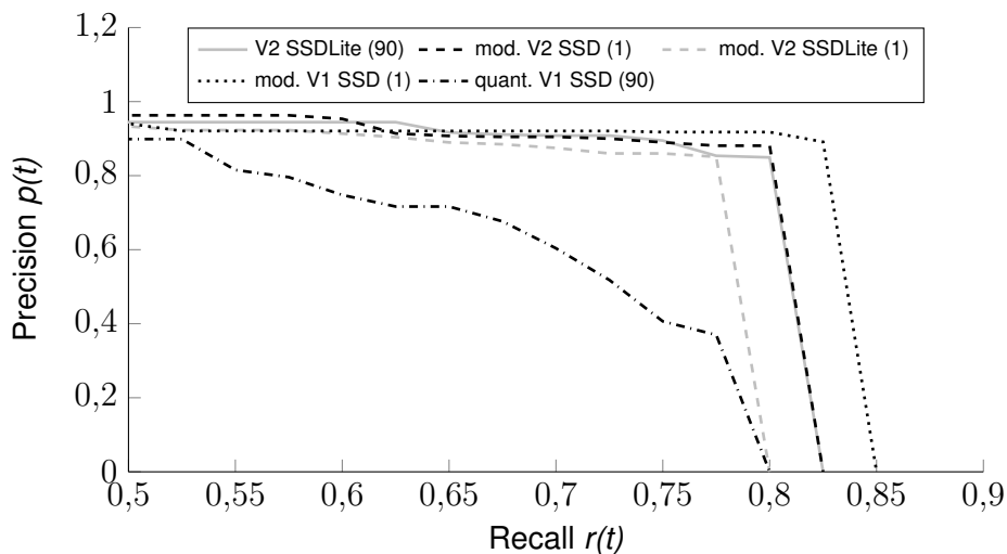
Abbildung 4.9: Precision-Recall Kurven aller MobileNet Architekturen in Anwendung auf den eigenen Datensatz. Die Abkürzungen mod. und quant. stehen für modifiziert und quantisiert .
